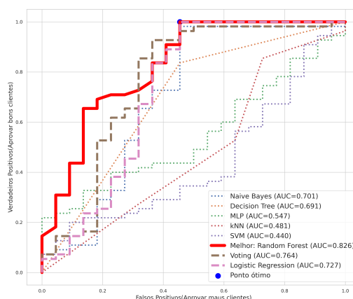
Figura 1. Curvas ROC dos modelos de classificação no conjunto de teste.
